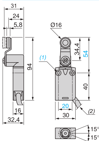
XCMD2●16L1
